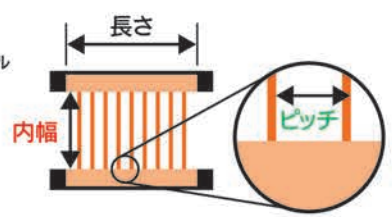
U字溝を上から見た図
