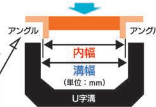
U字溝の断面から見た図
